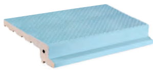
410 SOPORTE REJILLA DOTS 13,5X24,5X3,5 / 5,3"X9,6"X1,4" K87/P ONLY / SOLO: ● Azul, ● Perla, ● Beige y ● Blanco.
