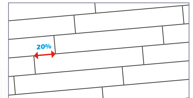
Colocación a matajuntas B. Recomendamos colocación trabada al 20%.
