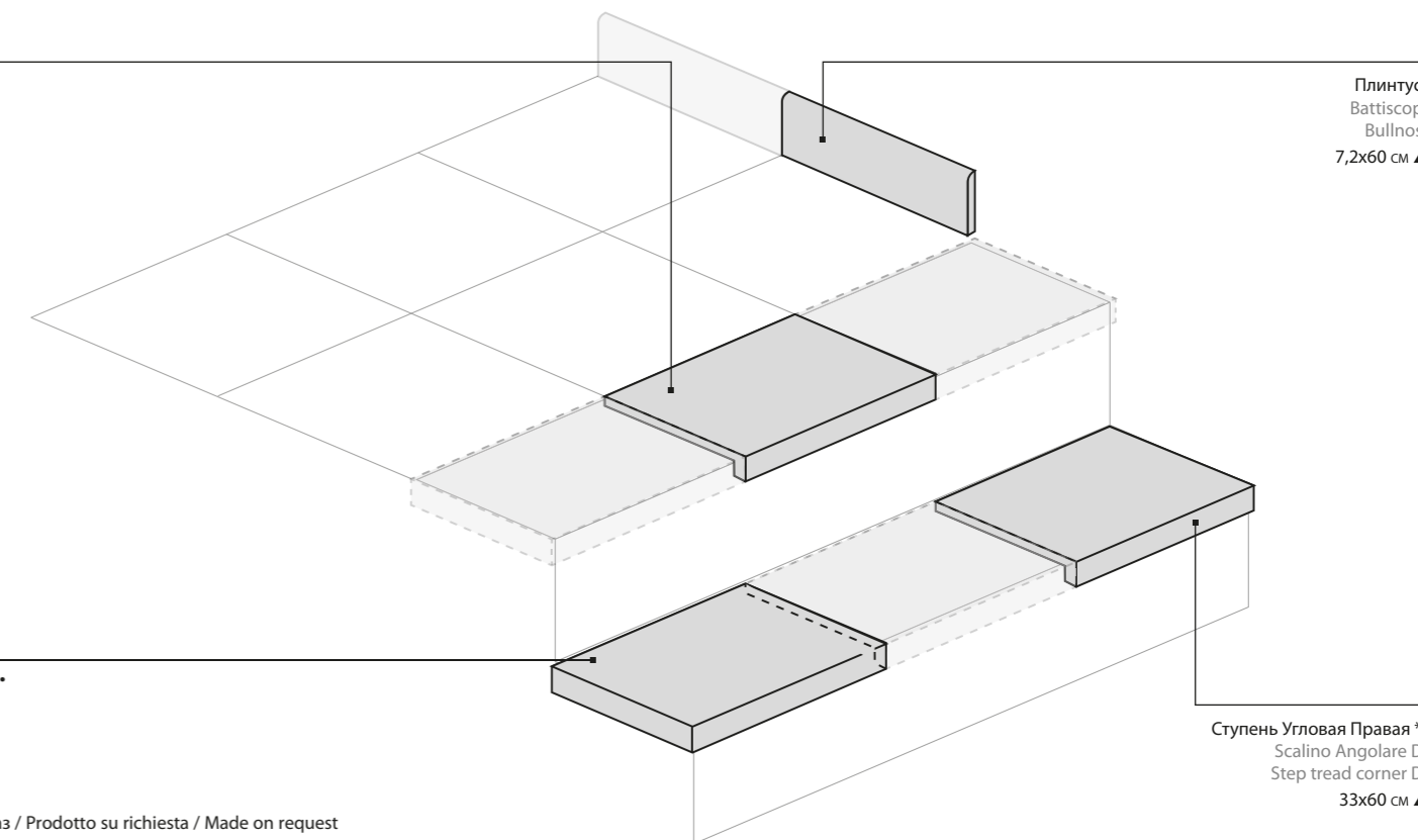
Ступень Фронтальная ** Scalino Frontale Step tread Front 33x60 см ▲
