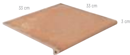
PELDAÑO FIORENTINO 33 x 33 x 3 cm - 13.0" x 13.0" x 1.2"
