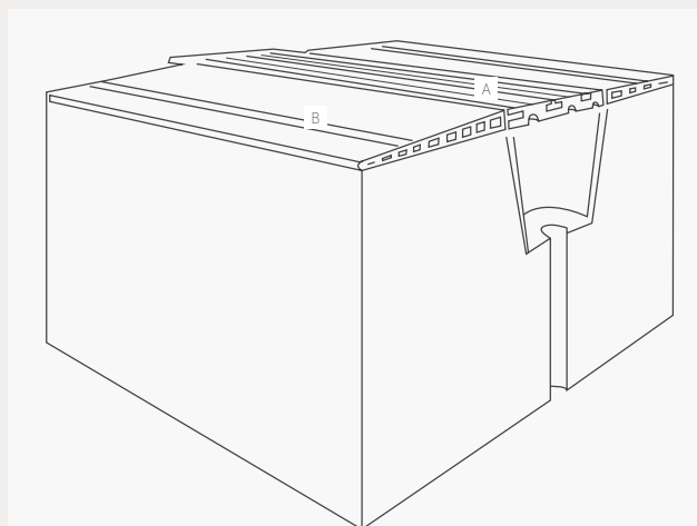
A - REJILLA 24,5 x 24,5 cm ( COLOCACIÓN ALTERNADA A 180° ) B - BORDE DESBORDANTE 28 x 66,5 cm C - REJILLA 24,5 x 24,5 cm ( COLOCACIÓN ALTERNADA A 180° ), VISTA CENITAL
